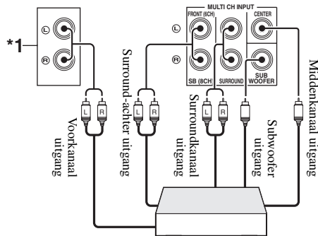
Multiformaat-speler/externe decoder (7.1-kanaals uitgangen)
