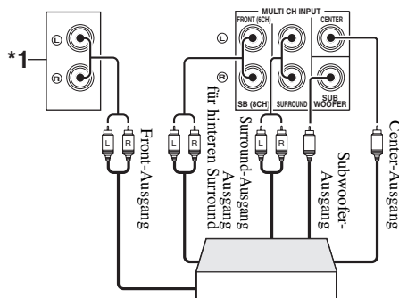
Multi-Format-Player/Etherner Decoder (7.1-Kanal-Ausgang)
