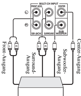
Multi-Format-Player/Etherner Decoder (5.1-Kanal-Ausgang)
