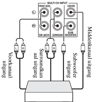
Multiformaat-speler/externe decoder (5.1-kanaals uitgangen)
