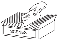
SCENE-Schablone-Bibliothek (Abbildung)
