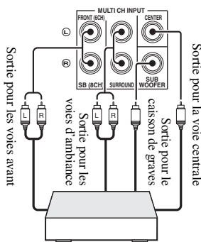
Lecteur multiformat/Décodeur extérieur (sortie 5.1 voies)
