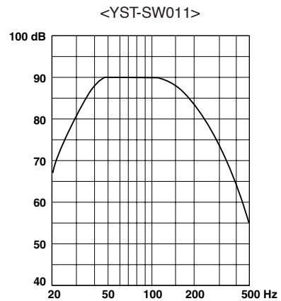
Diagram van de frequentiekenmerken*
