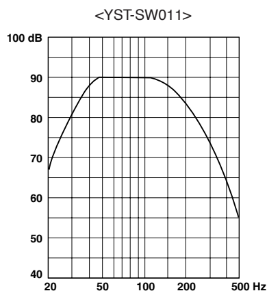
Grafico della risposta in frequenza*
